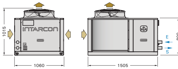
Dimensiones serie 1
