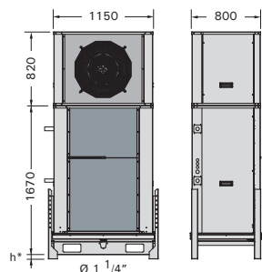
modelo 3256
