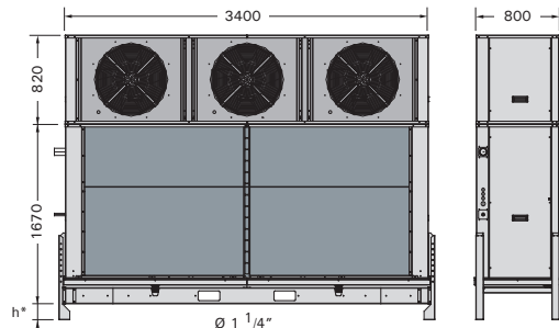
modelo 3363
