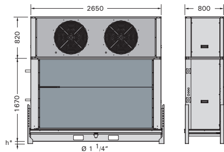
modelo 3363
